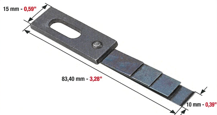
MOLLA (LINGUETTA SEPARAFOGLIO) SPRING (SHEET SEPARATOR) MOLLA (LENGÜETA SEPARADORA)
