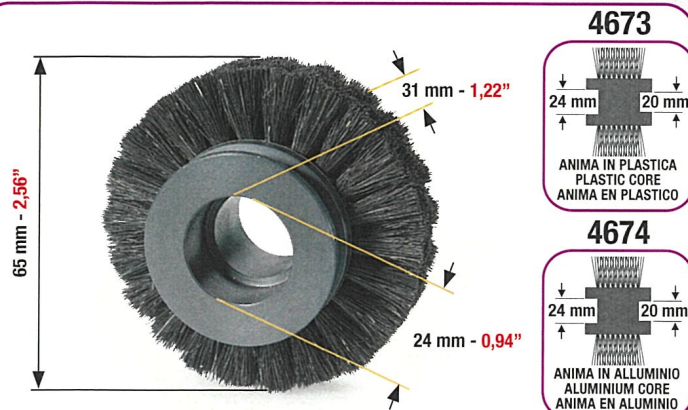
RUOTA A SPAZZOLA BRUSH WHEEL RUEDA DE CEPILLO
