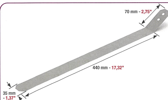
LAMA ABBATTI FOGLIO UNIVERSALE UNIVERSAL SHEET GUIDE GUIA DE LA HOJA UNIVERSAL
