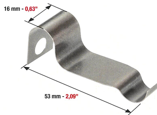
SEPARATORE CARTA SPRING SEPARATOR PAPER MUELLE SEPARADORA PAPEL
