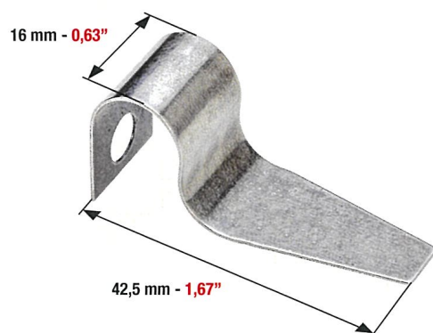
SEPARATORE FOGLI CARTONE SPRING SEPARATOR CARDBOARD MUELLE SEPARADORA CARTON
