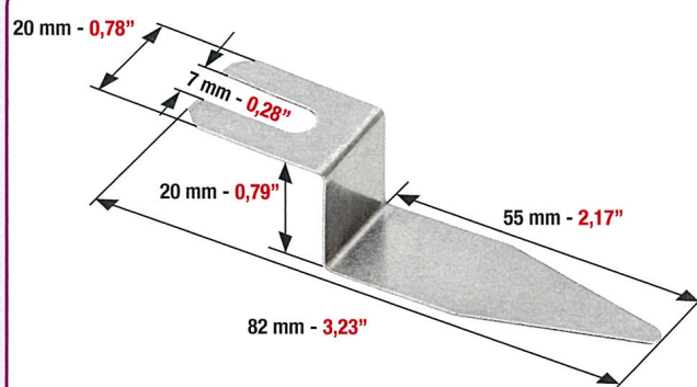
MOLLA (SEPARAFOGLIO PIATTA) SPRING (FLAT SEPARATOR) MUELLE (SEPARADORA PIANA)
