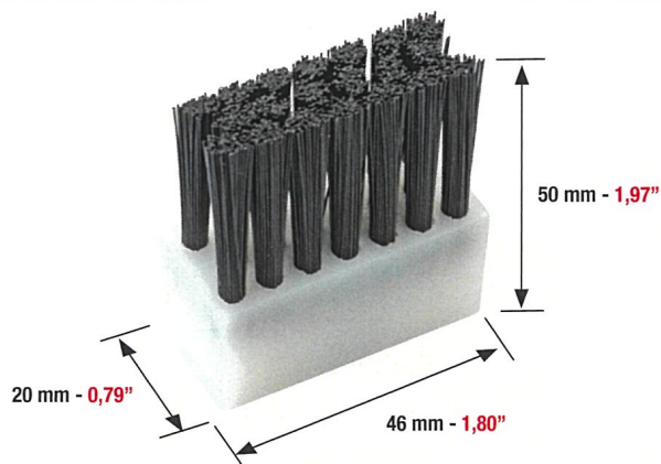
SPAZZOLA METTIFOGLIO CON PELO IN POLYAMIDE FEEDER BRUSH WITH POLYAMIDE BRISTLES CEPILLO PARA MARCADOR CON PELO DE POLYAMIDA
