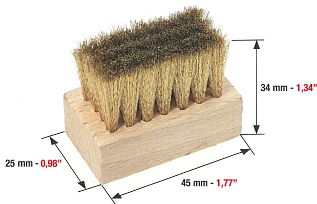
SPAZZOLINO CON PELO IN OTTONE FEEDER BRUSH WITH BRASS BRISTLES PEQUEÑO CEPILLO CON PELO DE LATÓN
