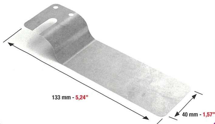
MOLLA (SEPARAFOGLIO PIATTA) BILATERALE CER-CER2 SPRING (FLAT SEPARATOR) BILATERAL CER-CER2 MUELLE (SEPARADORA PIANA) BILATERAL CER-CER2
