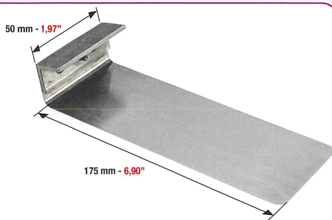
LAMA D'APPOGGIO (BATTIFOGLIO) - BOBST 142 SUPPORT BLADE (SHEET GUIDE) REGLETA DE SOPORTE
