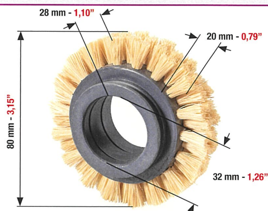
RUOTA A SPAZZOLA PER CARTONE ONDULATO BRUSH WHEEL FOR CORRUGATED CARDBOARD RUEDA DE CEPILLO PARA CARTON ONDULADO
