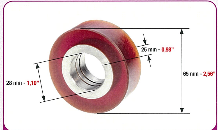
RUOTA DI INTRODUZIONE FOGLI PIANO DI PUNTATURA SHEET FEEDER WHEEL FOR ENTRY TABLE RUEDE DE INTRODUCCION DEL PLIEGO A LA MESA DE REGISTRO
