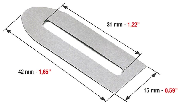
LINGUETTA PIATTA SPRING (FLAT) MOLLA (PLANA)
