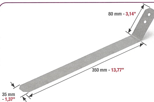
LAMA ABBATTI FOGLIO UNIVERSALE UNIVERSAL SHEET GUIDE GUIA DE LA HOJA UNIVERSAL
