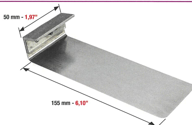
LAMA D'APPOGGIO (BATTIFOGLIO) - BOBST 142 SUPPORT BLADE (SHEET GUIDE) REGLETA DE SOPORTE
