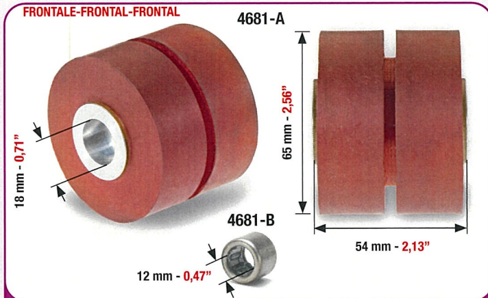
RUOTA DI TRASPORTO PER TAVOLA DI PUNTATURA (INTRODUZIONE) SHEET FEEDER WHEEL FOR ENTRY TABLE RUEDE DE TRANSPORTE PARA MESA DE REGISTRO (INTRODUCCION)
