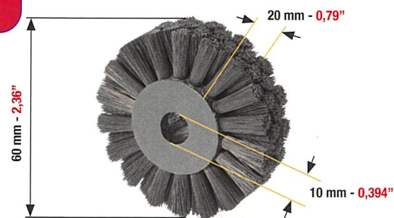
RUOTA A SPAZZOLA BRUSH WHEEL RUEDA DE CEPILLO
