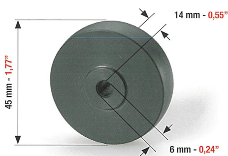
RUOTA DI TRASPORTO IN PLASTICA PER: FEEDER WHEEL IN PLASTIC FOR: RUEDA DE TRANSPORTE DE PLÁSTICO PARA:
