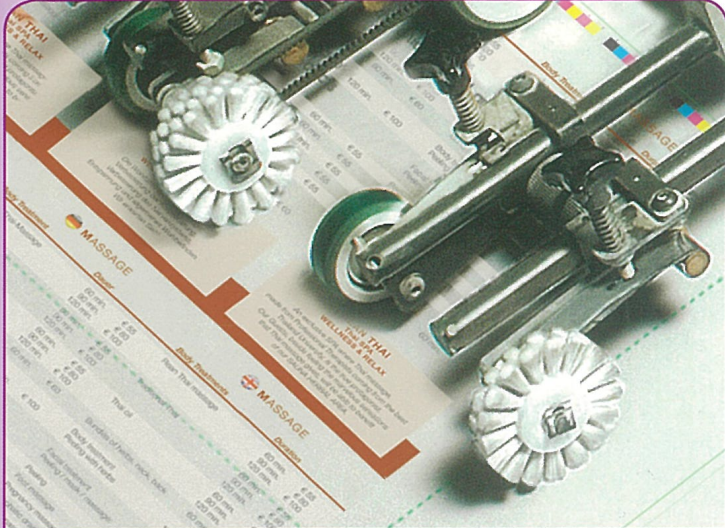
RUOTE DI TRASPORTO PER SEZIONE METTIFOGLIO FEEDER WHEELS RUEDAS DE TRANSPORTE PARA MARCADOR
