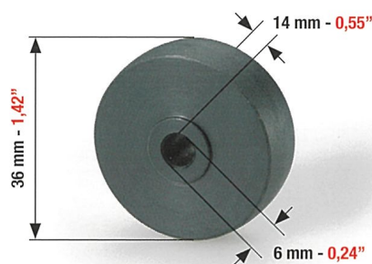
RUOTA DI TRASPORTO IN PLASTICA PER: FEEDER WHEEL IN PLASTIC FOR: RUEDA DE TRANSPORTE DE PLÁSTICO PARA:
