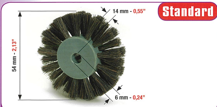
RUOTA DI TRASPORTO A SPAZZOLA PER: BRUSH WHEEL FOR: RUEDA DE CEPILLO PARA:
