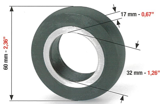
RUOTA DI TRASPORTO IN GOMMA PER: RUBBER WHEEL FOR FEEDER FOR: RUEDA DE TRANSPORTE EN GOMA PARA:
