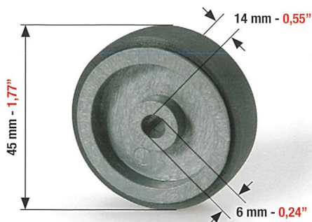
RUOTA DI TRASPORTO IN PLASTICA E GOMMA PER: FEEDER WHEEL IN PLASTIC AND RUBBER FOR: RUEDA DE TRANSPORTE DE PLÁSTICO Y GOMA PARA:
