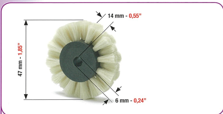
RUOTA BIANCA A SPAZZOLA PER CARTA PER: WHITE BRUSH WHEEL FOR PAPER FOR: RUEDA DE CEPILLO BLANCO PARA PAPEL PARA:
