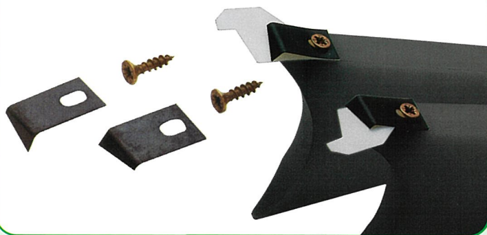
PIASTRINE BLOCCA RASCHIETTO COMPLETE DI VITI SCRAPER HOLDER PLATE COMPLETE WITH SCREWS PLACA FIJADORA DEL RASCADOR CON TORNILLO
