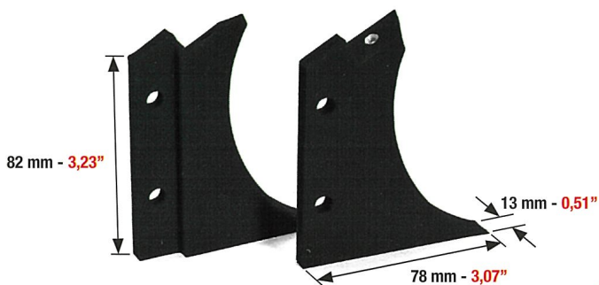
SPALLE DI BLOCCAGGIO COPRICALAMAIO PER: INK DUCT END BLOCKS FOR: RESPALDO DE BLOQUEO DEL CUBRETINTERO PARA:
